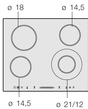
ET6..MN..D
