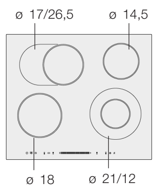
ET6..MN..D
