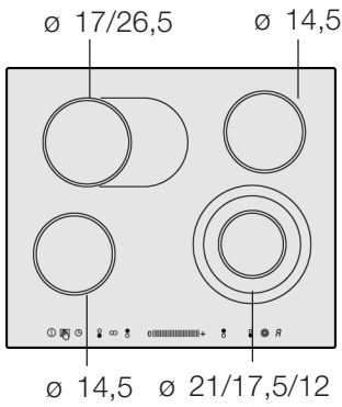
ET6..MD..
