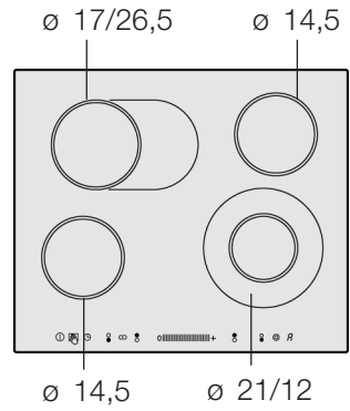
ET6..MN..
