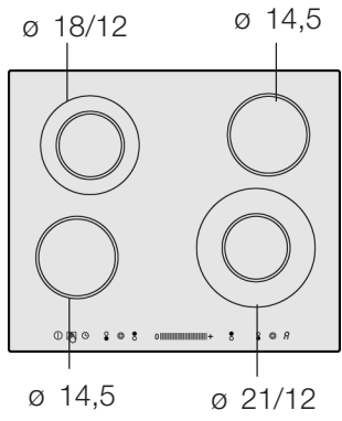
ET6..MK..
